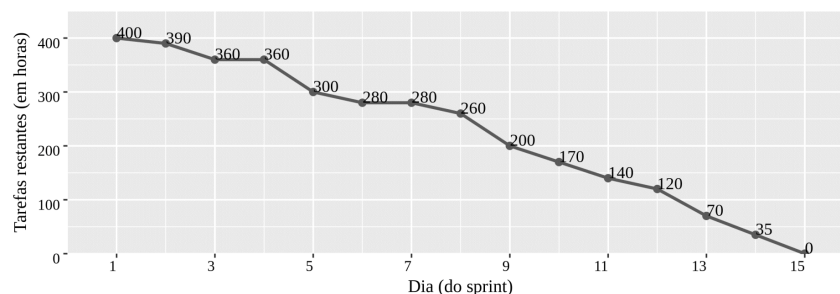
Gráfico de Burndown, assumindo um sprint com duração de 15 dias.
