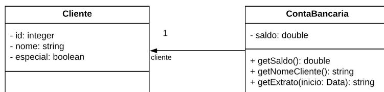
Exemplo de Diagrama de Classe UML com duas classes, Cliente e ContaBancaria .
