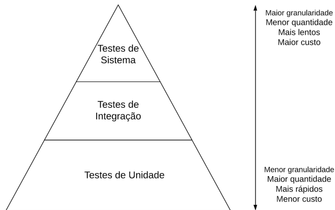
Pirâmide de testes
